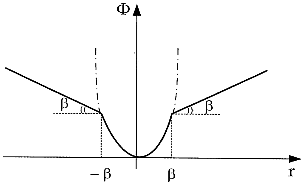
Fig. 1 – Huber Function
