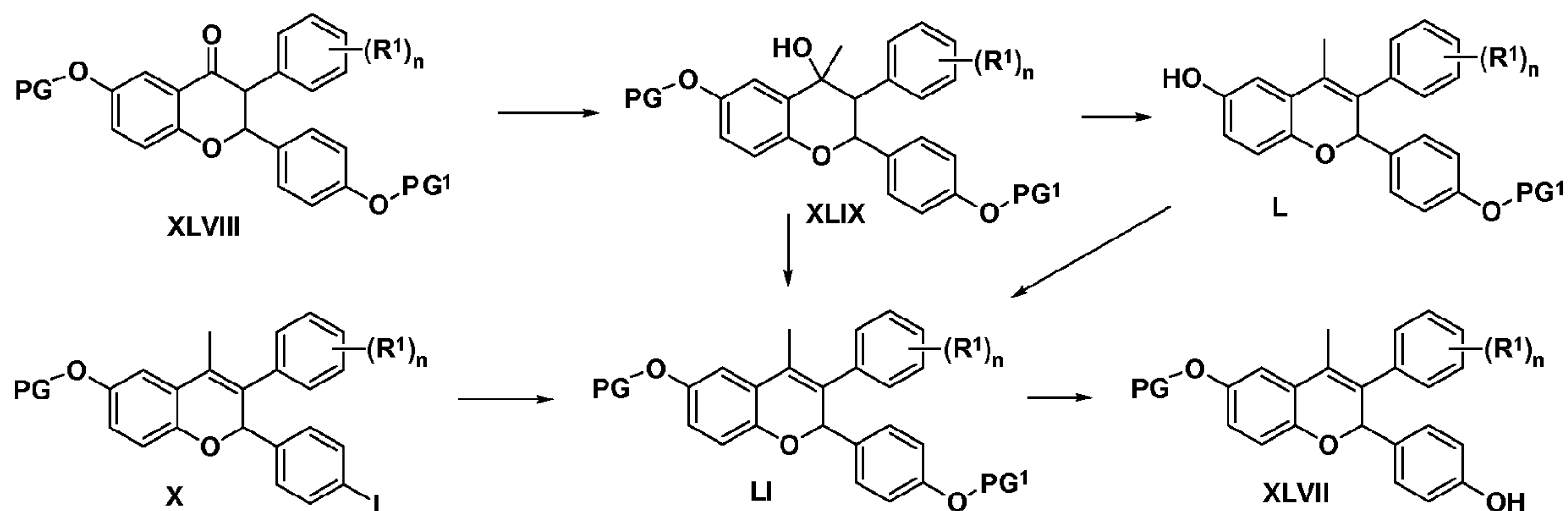
Scheme 14.
