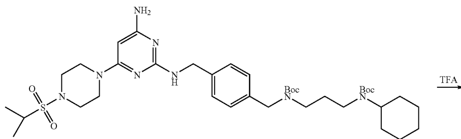
109-II
