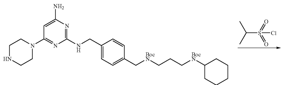
109-I
