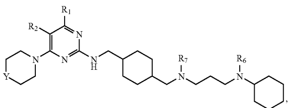
(XVIII)
