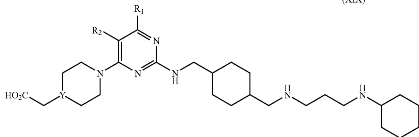
(XIX)
