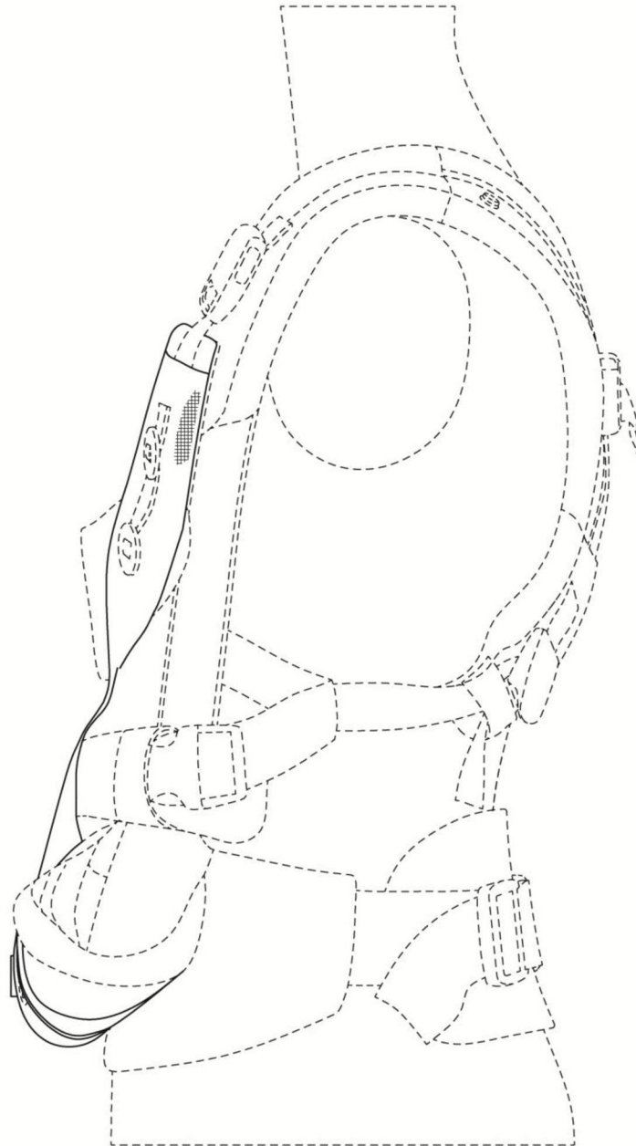
【右側視圖】
