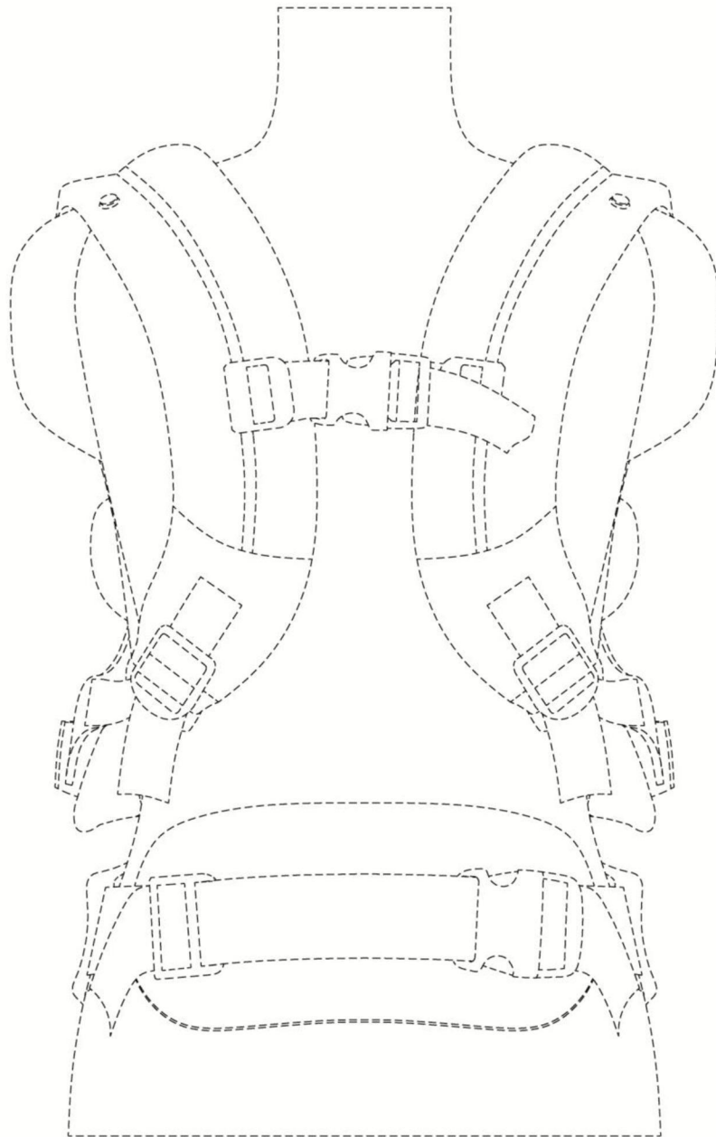
【後視圖】
