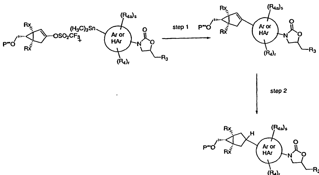
Scheme VI
