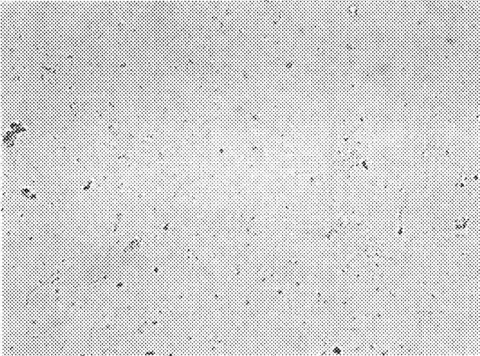
(+)-JQ1 50 mpk 8 weeks
