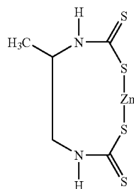
(ANTRACOL)
