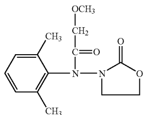
(OXADIXYL)
