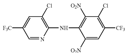
(FLUAZINAM)
