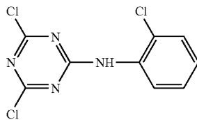
(ANILAZIN)
