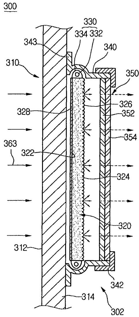
FIG. 13
