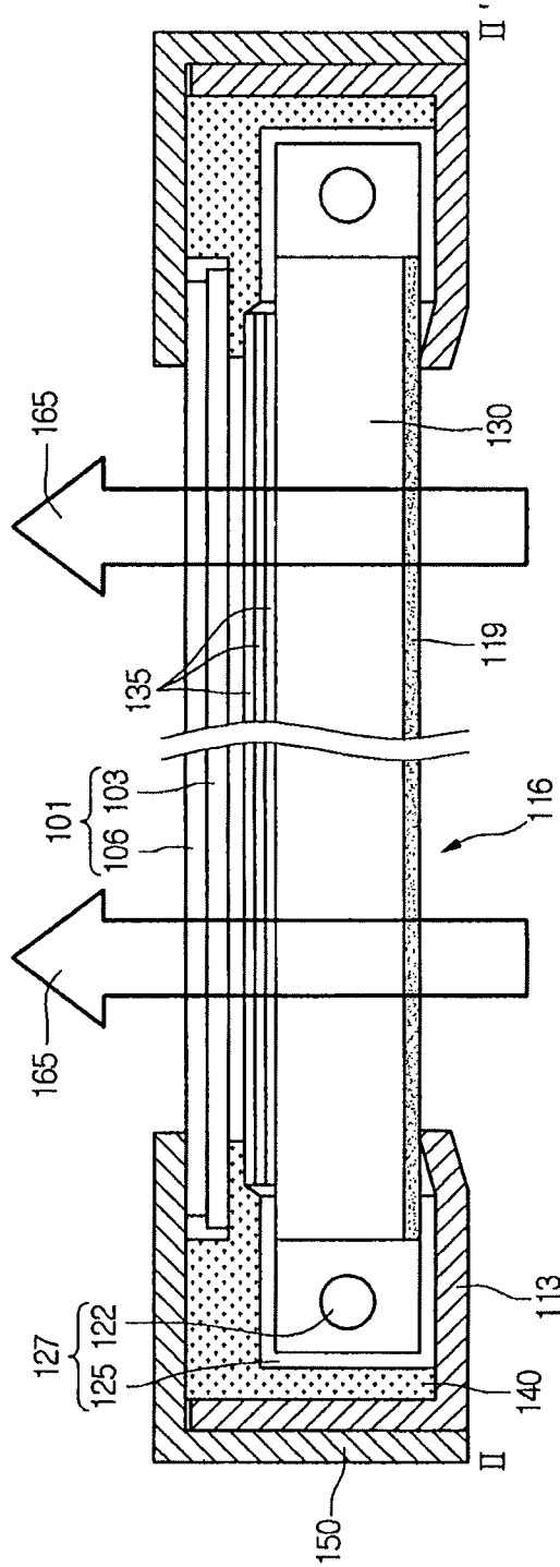
FIG. 4B
