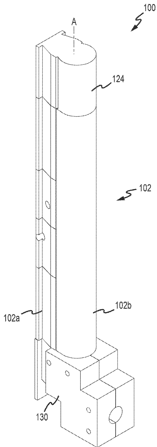
FIG. 1A
