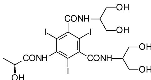
lopamidol
