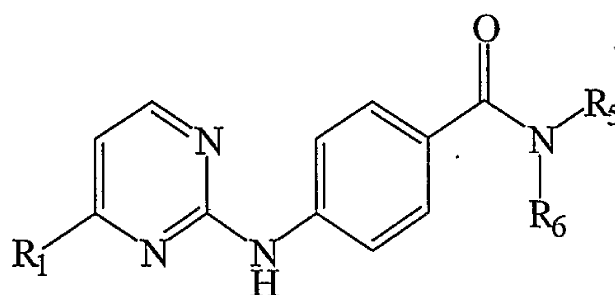
(IIA)
