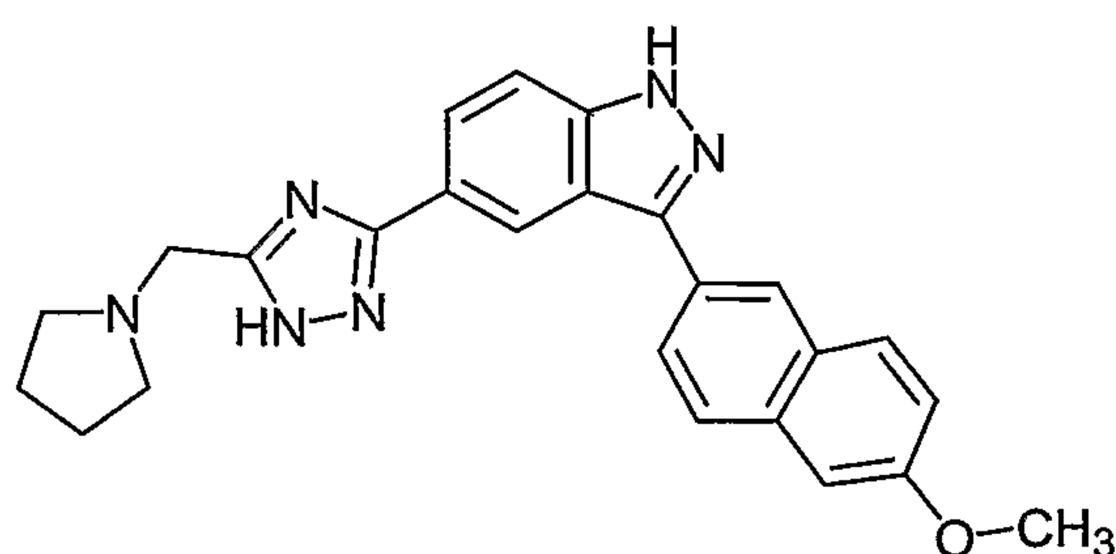
3-(6-Methoxy-naphthalen-2-yl)-5-(5-pyrrolidin-1-ylmethyl-1 H -[1,2,4]triazol-3-yl)-1 H -indazole ;
