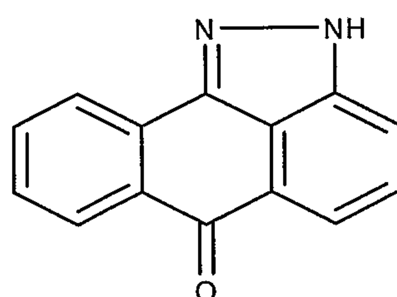
15 2H-Dibenzo[cd,g] indazol-6-one ;
