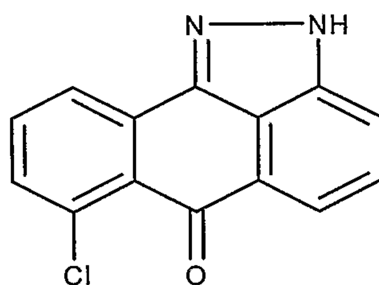
7-Chloro-2H-dibenzo[cd,g] indazol-6-one ;
