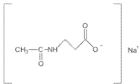
Sodium N-acetyl-beta-alaninate
