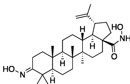
3-Oxo-lup-20(29)-en-28-acid
