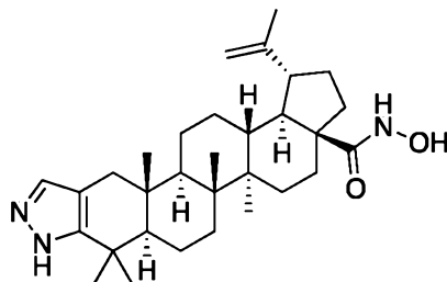
1'H-Lup-20(29)-eno[3,2-c]pyrazol-N-hydroxy-28-amide
