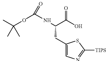
(S)-methyl 2-(tert-butoxycarbonyl)-3-(2-(triisopropylsilyl)thiazol-5-yl)propanoate
