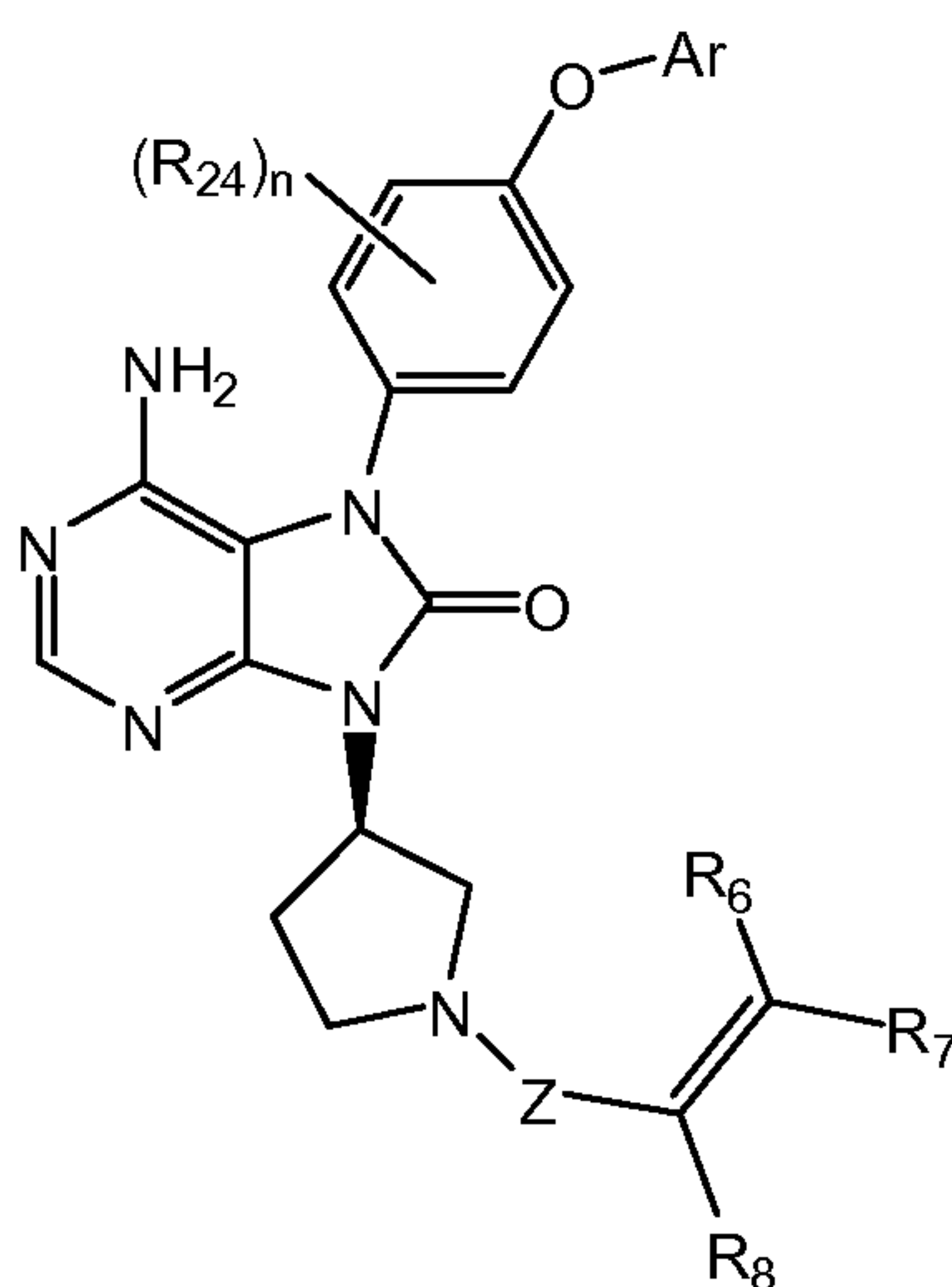
Formula (IIa);
