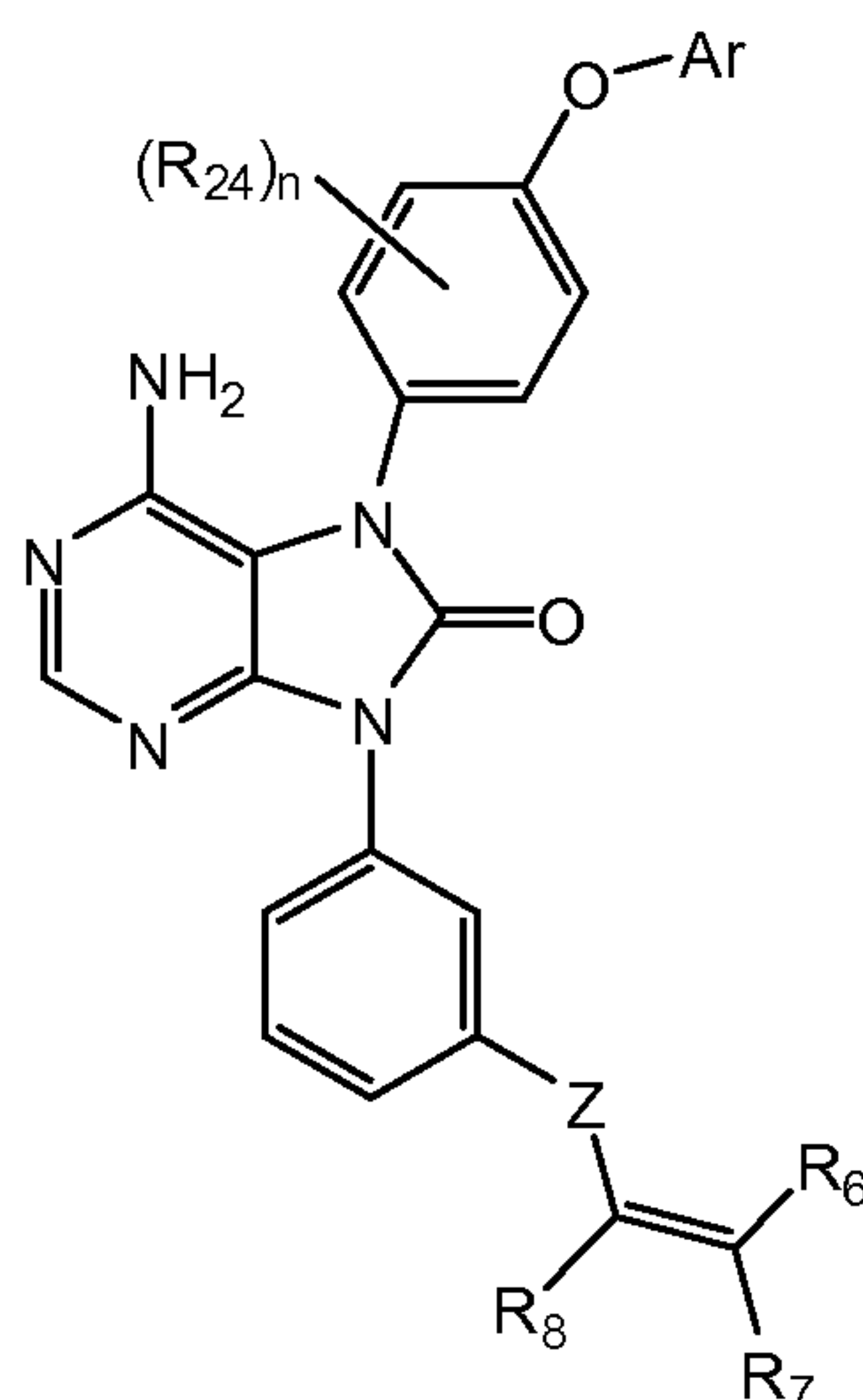
Formula (Ia);
