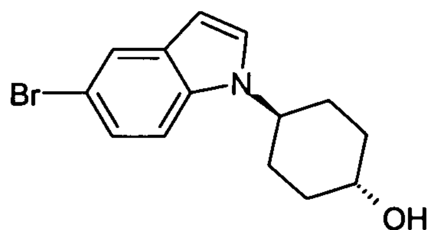
trans-D13
