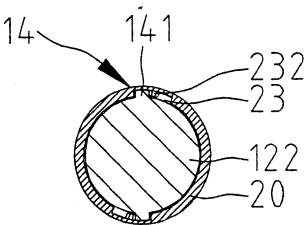
圖 十一B 11B-11B
