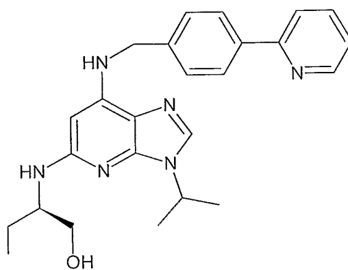
Formula Ic
