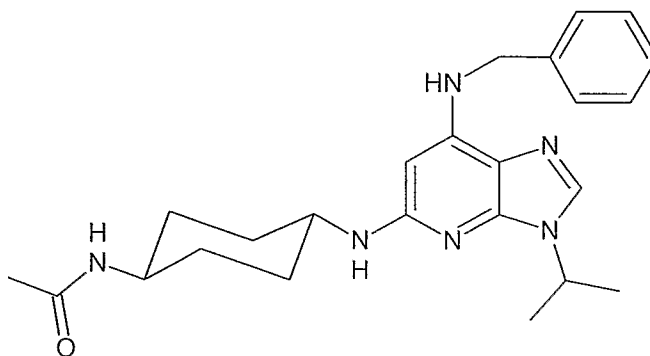
Formula Ih.
