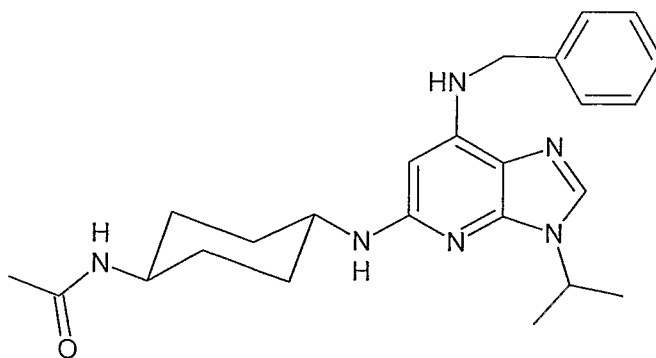
Formula Ih.
