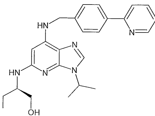
Formula Ic
