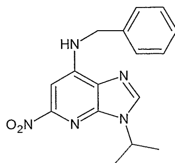
Formula 1e
