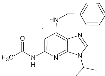
Formula Ig.
