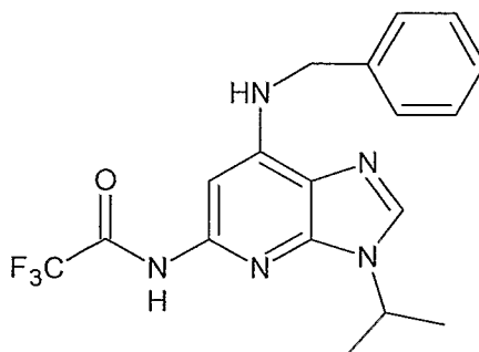
Formula Ig.
