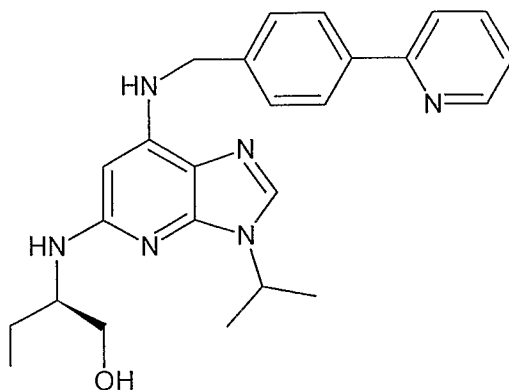
Formula Ic
