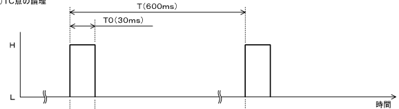
(b) TB点の出力電流の波形
