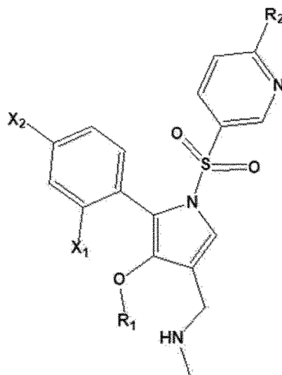
[Formule chimique 2]
