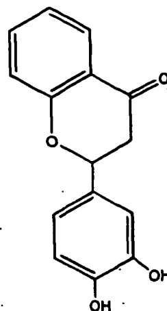
Flavanone (10)
