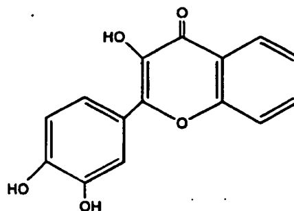
Flavonol (16)
