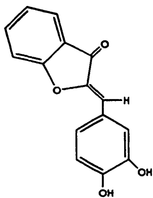
Aurone (14)
