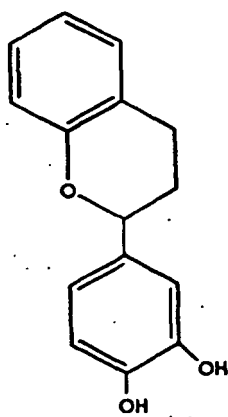
Flavan (12)
