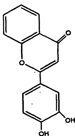
Flavone (8)
