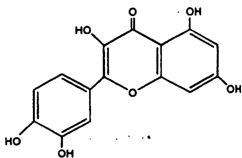
Quercetin (17)
