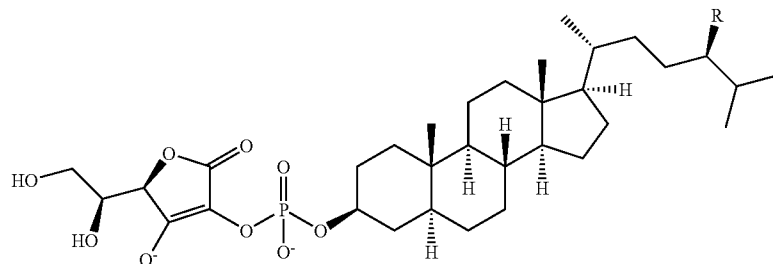
R = CH 3 ; CH 2 —CH 3 FM-VP4
