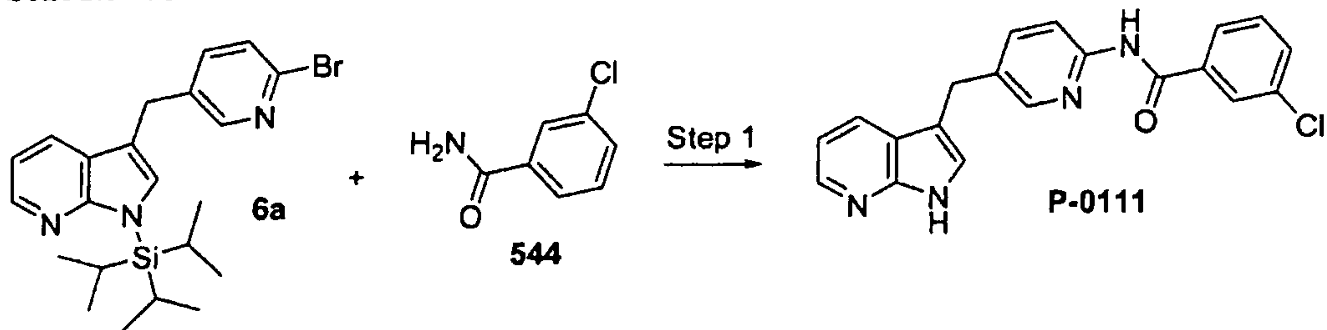
Scheme 170
