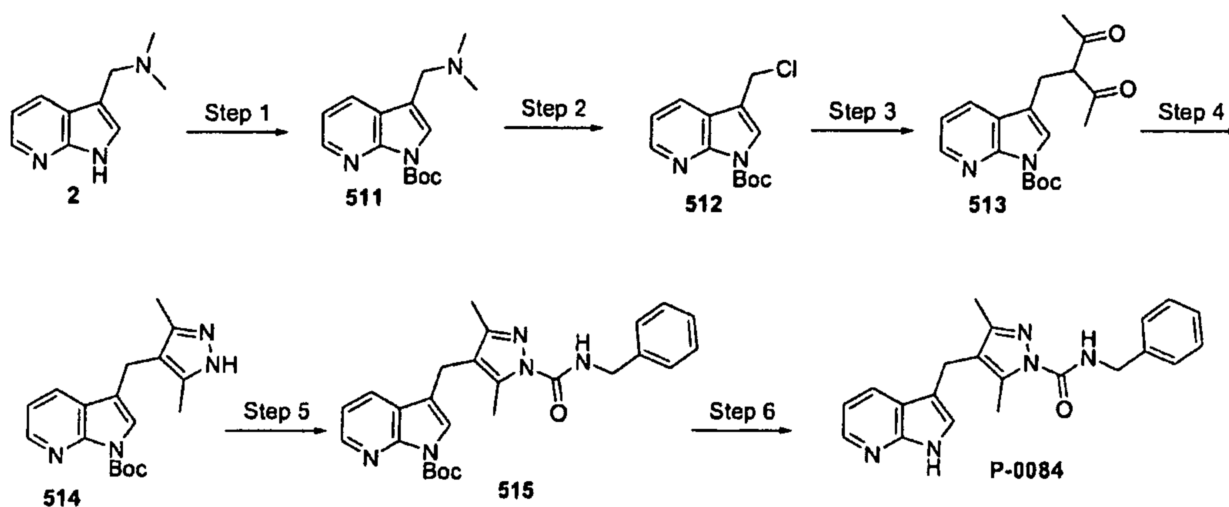
Scheme – 158
