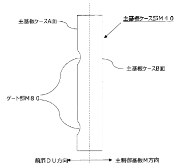
&lt;主基板ケースの側面図&gt;
