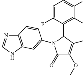
1-(1H-Benzo[d]imidazol-6-yl)-5-(2-chloro-3,6-difluorophenyl)-3-methoxy-4-methyl-1H-pyrrol-2(5H)-one;
