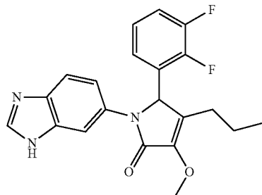
1-(1H-Benzo[d]imidazol-6-yl)-5-(2,3-difluorophenyl)-3-methoxy-4-propyl-1H-pyrrol-2(5H)-one;
