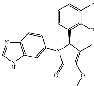
(R)-1-(1H-Benzo[d]imidazol-6-yl)-5-(2,3-difluorophenyl)-3-methoxy-4-methyl-1H-pyrrol-2(5H)-one;
