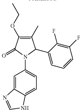
1-(1H-benzo[d]imidazol-5-yl)-3-ethoxy-5-(2,3-difluorophenyl)-4-methyl-1H-pyrrol-2(5H)-one;
