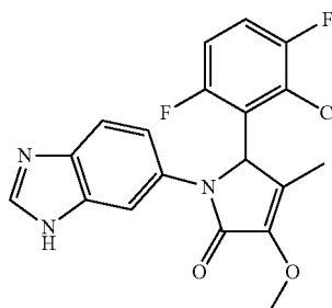
1-(1H-Benzo[d]imidazol-6-yl)-5-(2-chloro-3,6-difluorophenyl)-3-methoxy-4-methyl-1H-pyrrol-2(5H)-one;
