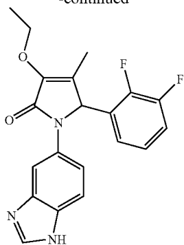
1-(1H-Benzo[d]imidazol-5-yl)-3-ethoxy-5-(2,3-difluorophenyl)-4-methyl-1H-pyrrol-2(5H)-one;
