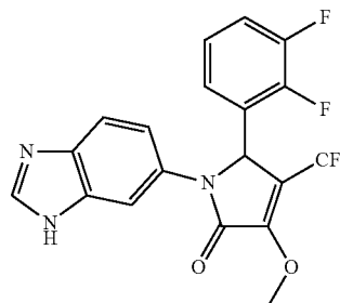
1-(1H-Benzo[d]imidazol-6-yl)-4-(trifluoromethyl)-5-(2,3-difluorophenyl)-3-methoxy-1H-pyrrol-2(5H)-one;
