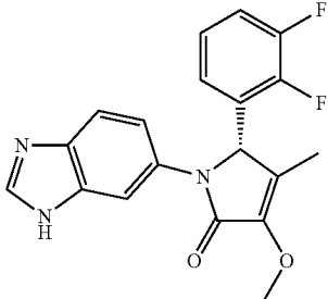
(S)-1-(1H-Benzo[d]imidazol-6-yl)-5-(2,3-difluorophenyl)-3-methoxy-4-methyl-1H-pyrrol-2(5H)-one;
