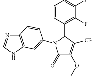
1-(1H-Benzo[d]imidazol-6-yl)-4-(trifluoromethyl)-5-(2,3-difluorophenyl)-3-methoxy-1H-pyrrol-2(5H)-one;
