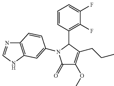
1-(1H-Benzo[d]imidazol-6-yl)-5-(2,3-difluorophenyl)-3-methoxy-4-propyl-1H-pyrrol-2(5H)-one;
