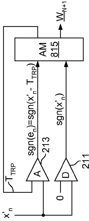
FIG. 30
