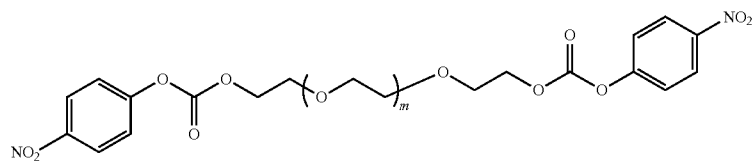
PEG—DiNPC (MW = 3400 Da)
