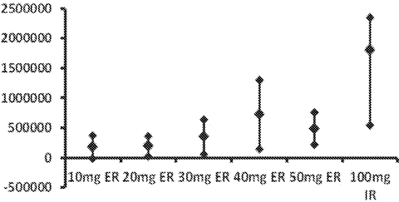
Onapristone AUC vs Dose
