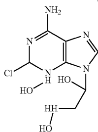
Cladridine
