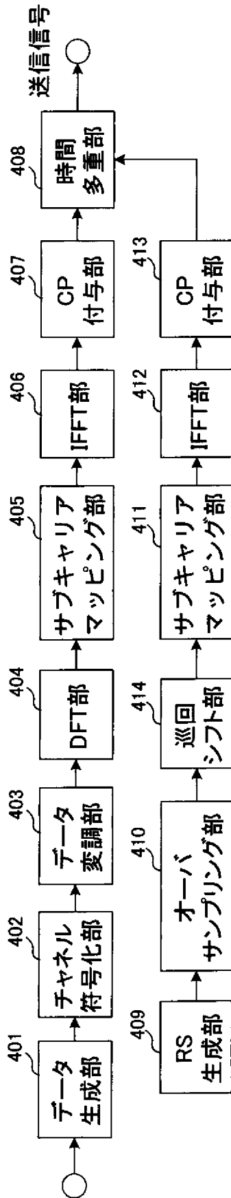
図18A 送信機
