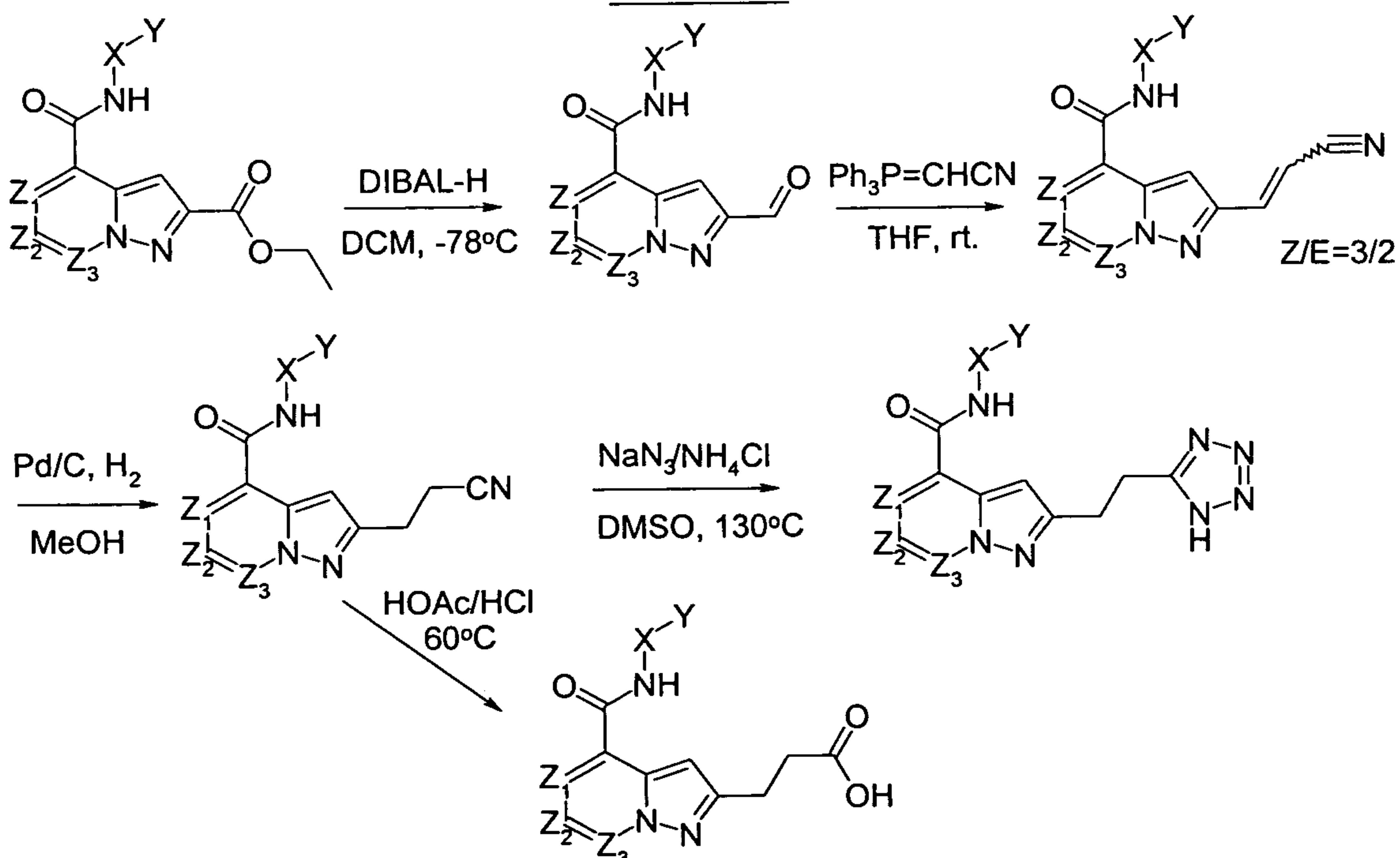
Scheme VI
