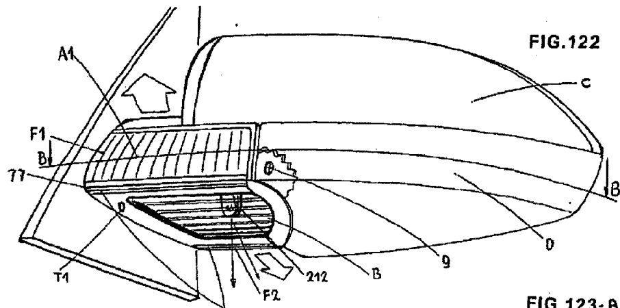
FIG. 123-A SECTION B-B
