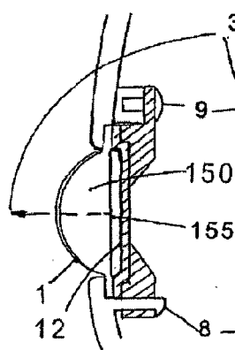
FIG.73A SECTION A-A
