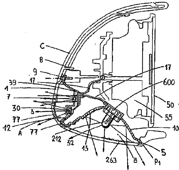
FIG.115 SECTION A-A
