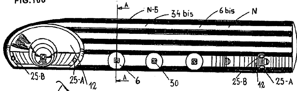
FIG.107 SECTION A-A
