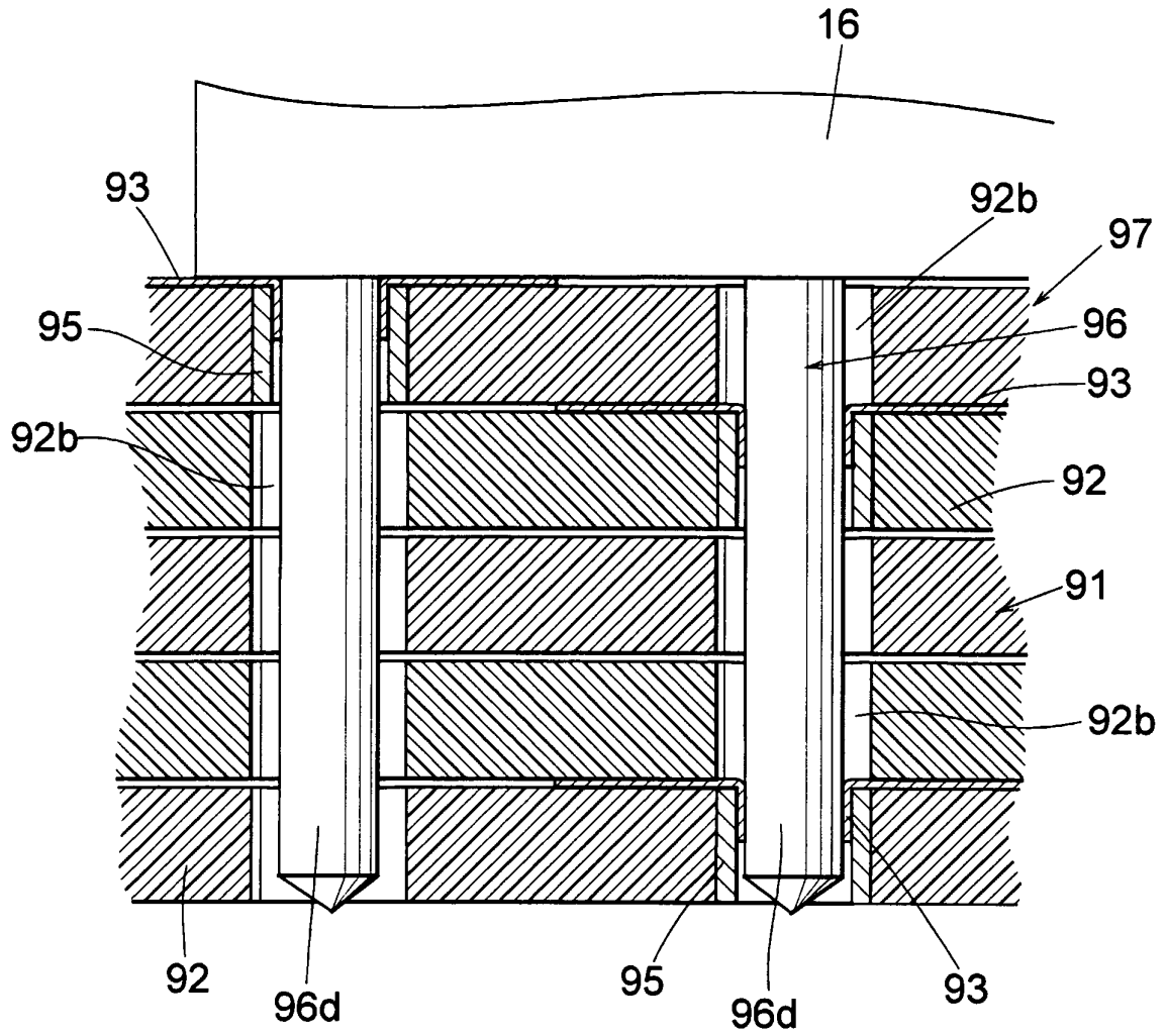
Fig. 27
