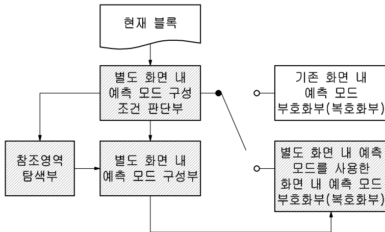
(b) 추가 시그널링 없는 본 발명의 세부 장치도
