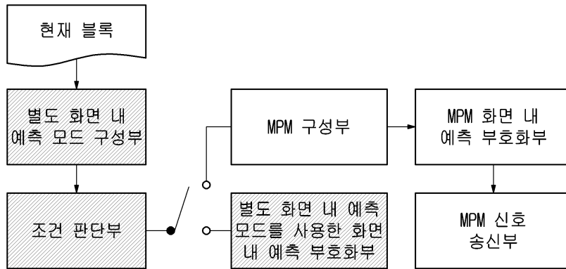
(a) 별도 화면 내 예측 모드를 사용한 부호화 장치
