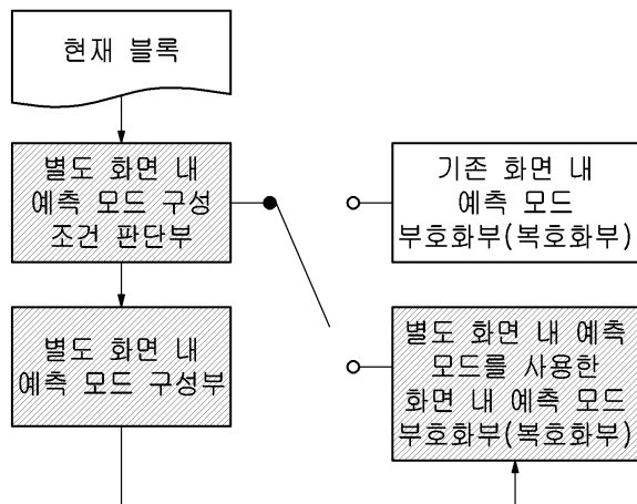
(b) 추가 시그널링 없는 본 발명의 세부 장치도
