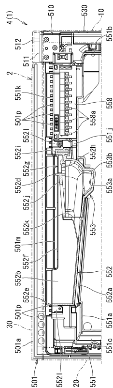
B-B断面图
