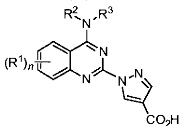
Formule (I)
