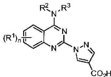
Formule (I)
