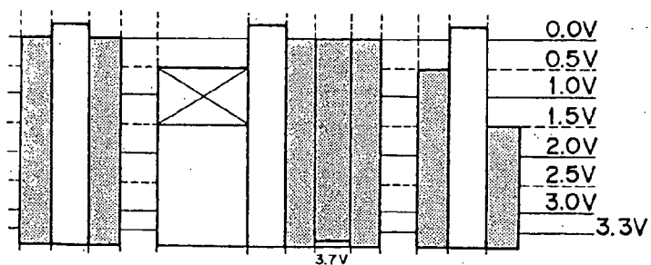
FIG. 15D t_3 < t < t_4
