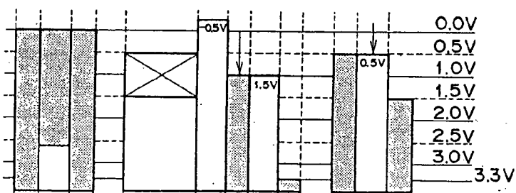
FIG. 13C t_2 < t < t_3 FD RESET
