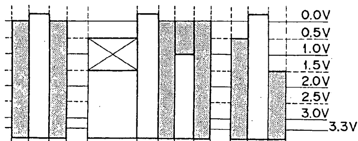
FIG. 16C t_7 < t
