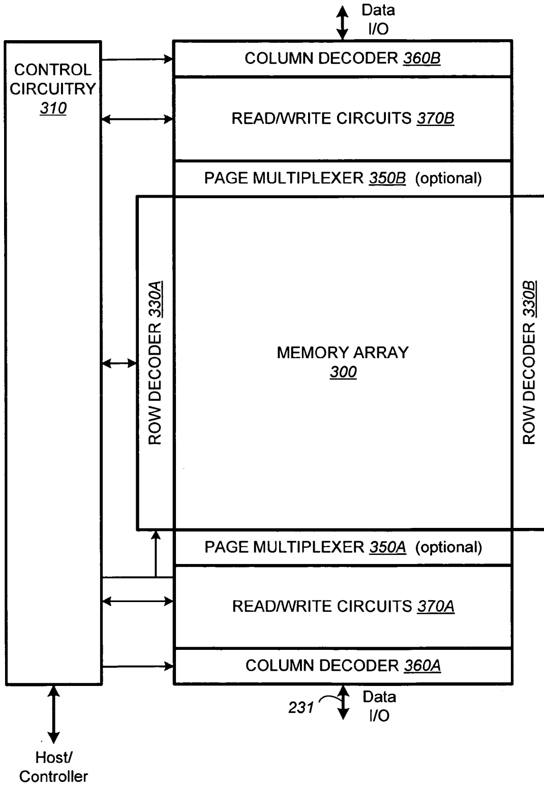
FIG. 6B
