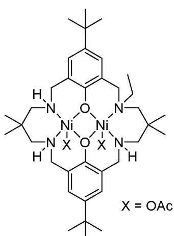
L^2Ni_2(OAc)_2
