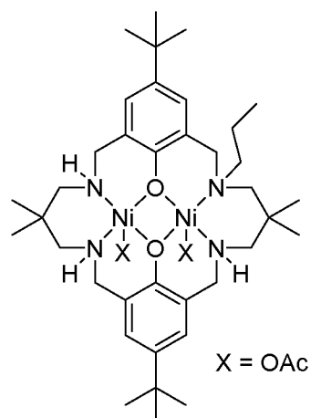
L^3Ni_2(OAc)_2
