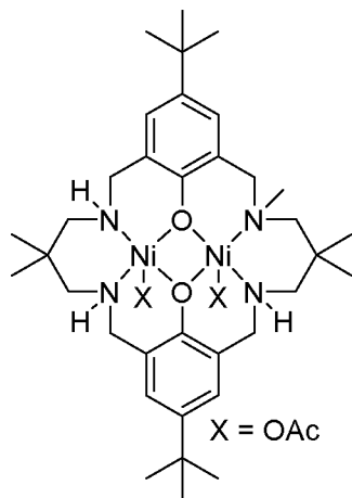
L^1Ni_2(OAc)_2
