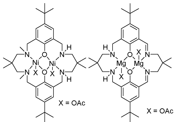
L^7Ni_2(OAc)_2
