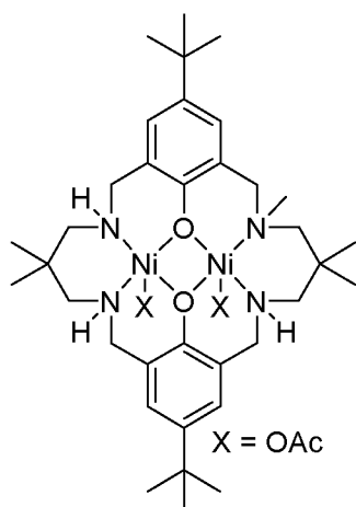
L^1Ni_2(OAc)_2
