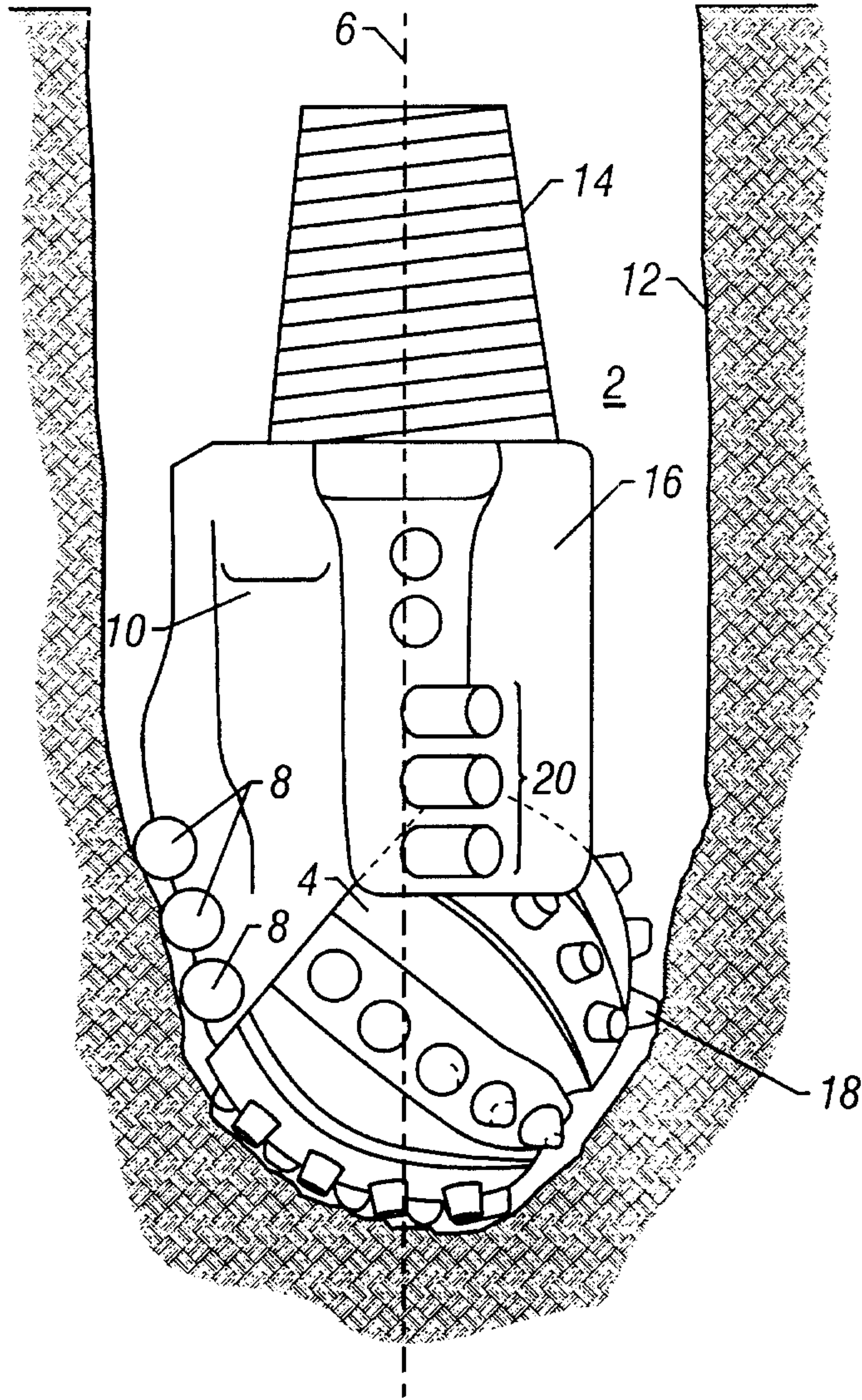
FIG. 4
