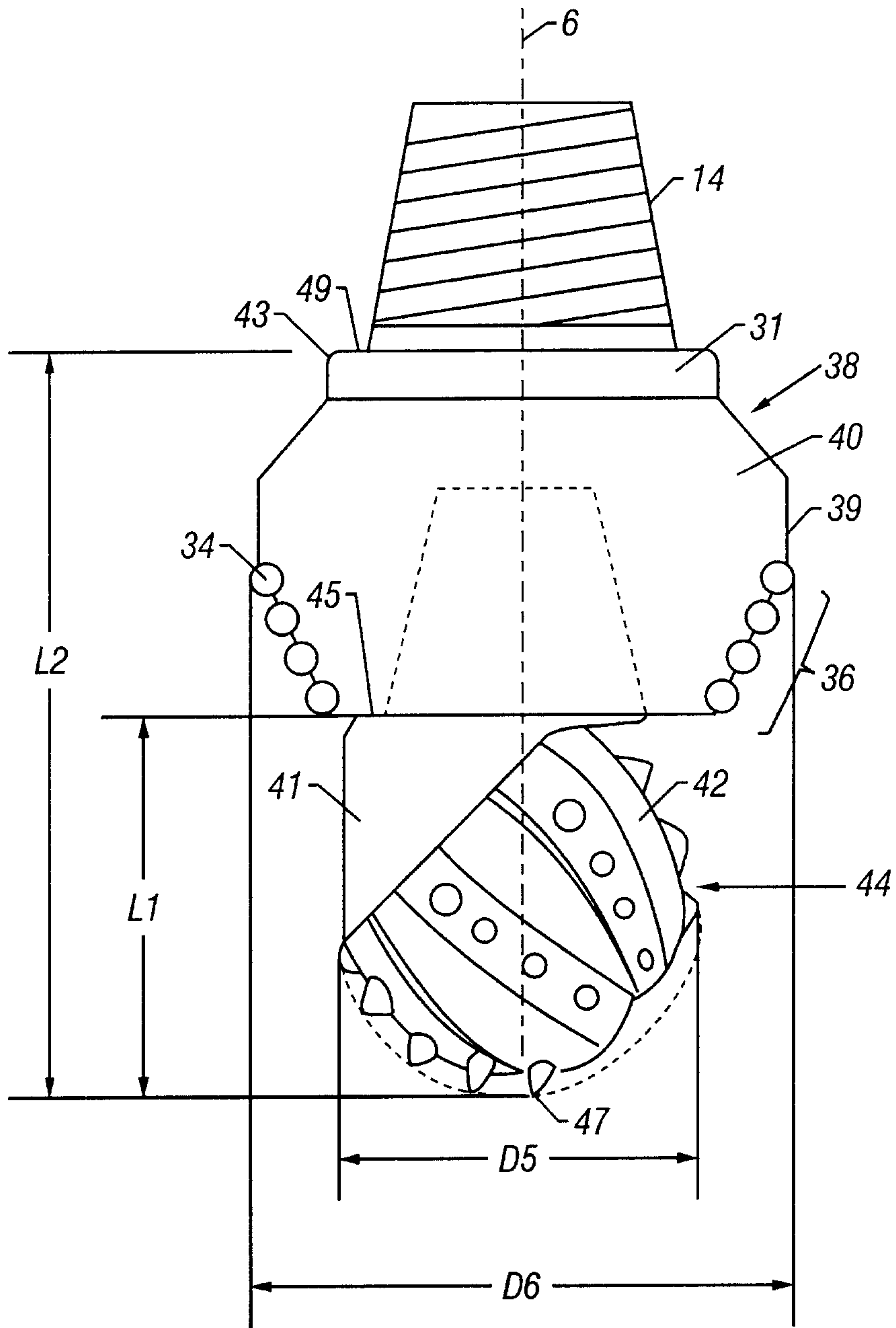
FIG. 7
