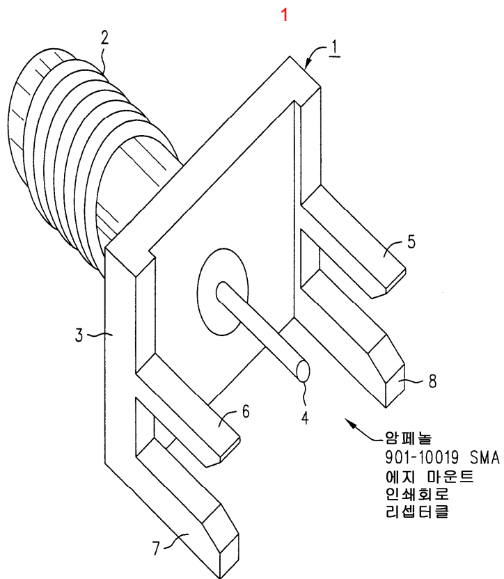
종래의 상업용 동축 RF 커넥터
