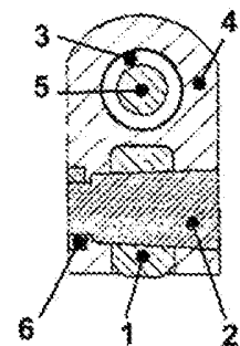
SECȚIUNEA B-B
