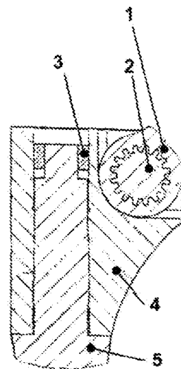
DETALIU C
