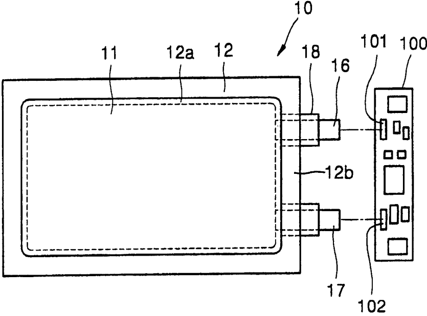
图 1 现有技术
