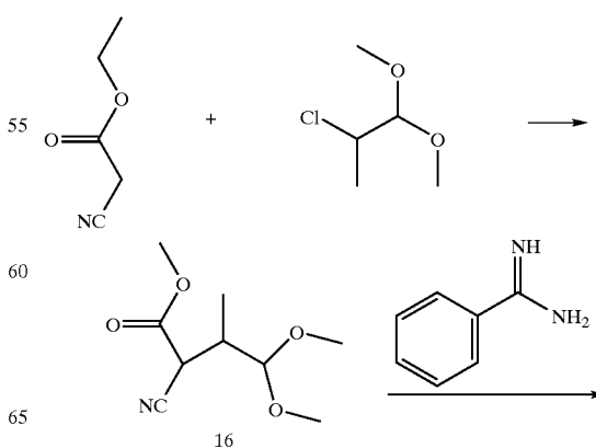
Scheme VI
