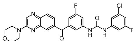
1-(3-chloro-5-fluorophenyl)-3-(3-fluoro-5-(3-morpholinoquinoxaline-6-carbonyl)phenyl)urea
