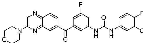
1-(3-chloro-4-fluorophenyl)-3-(3-fluoro-5-(3-morpholinoquinoxaline-6-carbonyl)phenyl)urea
