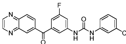
1-(3-chlorophenyl)-3-(3-fluoro-5-(quinoxaline-6-carbonyl)phenyl)urea
