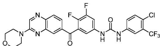
1-(4-chloro-3-(trifluoromethyl)phenyl)-3-(3,4-difluoro-5-(3-morpholinoquinoxaline-6-carbonyl)phenyl)urea
