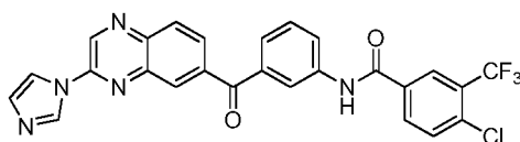
N -(3-(3-(1 H -imidazol-1-yl)quinoxaline-6-carbonyl)phenyl)-4-chloro-3-(trifluoromethyl)benzamide
