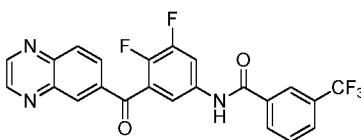
N-(3,4-difluoro-5-(quinoxaline-6-carbonyl)phenyl)-3-(trifluoromethyl)benzamide
