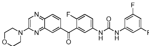
1-(3,5-difluorophenyl)-3-(4-fluoro-3-(3-morpholinoquinoxaline-6-carbonyl)phenyl)urea
