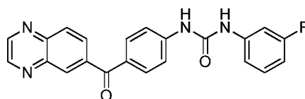
1-(3-fluorophenyl)-3-(4-(quinoxaline-6-carbonyl)phenyl)urea
