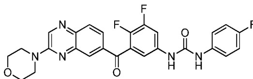
1-(3,4-difluoro-5-(3-morpholinoquinoxaline-6-carbonyl)phenyl)-3-(4-fluorophenyl)urea
