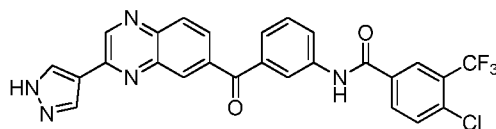
N-(3-(3-(1H-pyrazol-4-yl)quinoxaline-6-carbonyl)phenyl)-4-chloro-3-(trifluoromethyl)benzamide
