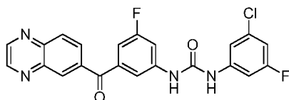
1-(3-chloro-5-fluorophenyl)-3-(3-fluoro-5-(quinoxaline-6-carbonyl)phenyl)urea
