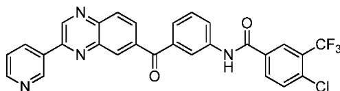
4-chloro- N -(3-(3-(pyridin-3-yl)quinoxaline-6-carbonyl)phenyl)-3-(trifluoromethyl)benzamide
