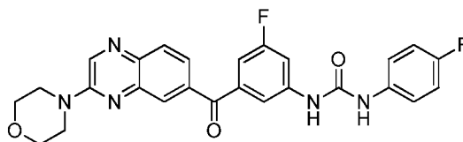
1-(3-fluoro-5-(3-morpholinoquinoxaline-6-carbonyl)phenyl)-3-(4-fluorophenyl)urea
