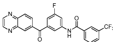
N-(3-fluoro-5-(quinoxaline-6-carbonyl)phenyl)-3-(trifluoromethyl)benzamide
