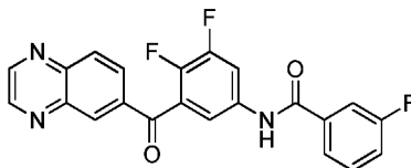
N-(3,4-difluoro-5-(quinoxaline-6-carbonyl)phenyl)-3-fluorobenzamide
