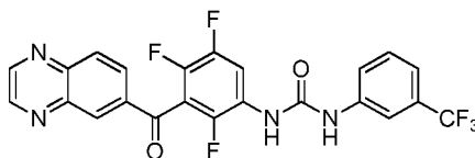
1-(2,4,5-trifluoro-3-(quinoxaline-6-carbonyl)phenyl)-3-(3-(trifluoromethyl)phenyl)urea
