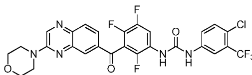
1-(4-chloro-3-(trifluoromethyl)phenyl)-3-(2,4,5-trifluoro-3-(3-morpholinoquinoxaline-6-carbonyl)phenyl)urea
