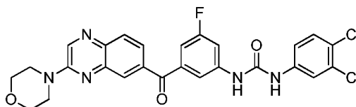
1-(3,4-dichlorophenyl)-3-(3-fluoro-5-(3-morpholinoquinoxaline-6-carbonyl)phenyl)urea
