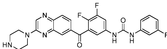
1-(3,4-difluoro-5-(3-(piperazin-1-yl)quinoxaline-6-carbonyl)phenyl)-3-(3-fluorophenyl)urea
