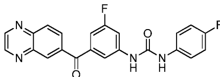
1-(3-fluoro-5-(quinoxaline-6-carbonyl)phenyl)-3-(4-fluorophenyl)urea
