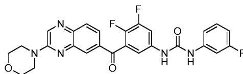
1-(3,4-difluoro-5-(3-morpholinoquinoxaline-6-carbonyl)phenyl)-3-(3-fluorophenyl)urea
