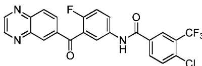
4-chloro-N-(4-fluoro-3-(quinoxaline-6-carbonyl)phenyl)-3-(trifluoromethyl)benzamide
