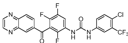
1-(4-chloro-3-(trifluoromethyl)phenyl)-3-(2,4,5-trifluoro-3-(quinoxaline-6-carbonyl)phenyl)urea
