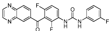
1-(2,4-difluoro-3-(quinoxaline-6-carbonyl)phenyl)-3-(3-fluorophenyl)urea
