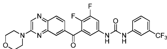
1-(3,4-difluoro-5-(3-morpholinoquinoxaline-6-carbonyl)phenyl)-3-(3-(trifluoromethyl)phenyl)urea
