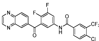
4-chloro-N-(3,4-difluoro-5-(quinoxaline-6-carbonyl)phenyl)-3-(trifluoromethyl)benzamide
