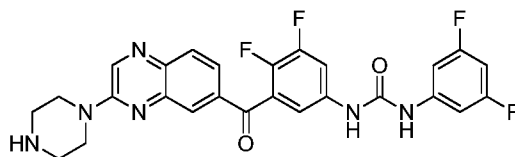
1-(3,4-difluoro-5-(3-(piperazin-1-yl)quinoxaline-6-carbonyl)phenyl)-3-(3,5-difluorophenyl)urea
