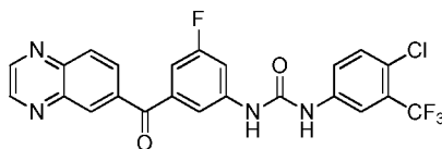
1-(4-chloro-3-(trifluoromethyl)phenyl)-3-(3-fluoro-5-(quinoxaline-6-carbonyl)phenyl)urea
