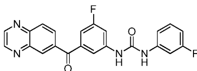
1-(3-fluoro-5-(quinoxaline-6-carbonyl)phenyl)-3-(3-fluorophenyl)urea
