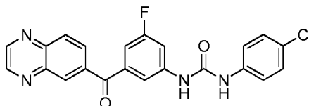
1-(4-chlorophenyl)-3-(3-fluoro-5-(quinoxaline-6-carbonyl)phenyl)urea
