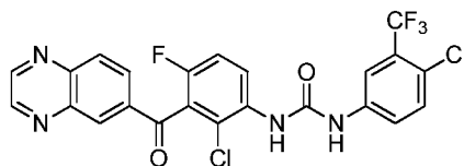
1-(4-chloro-3-(trifluoromethyl)phenyl)-3-(2-chloro-4-fluoro-3-(quinoxaline-6-carbonyl)phenyl)urea
