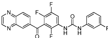
1-(3-fluorophenyl)-3-(2,4,5-trifluoro-3-(quinoxaline-6-carbonyl)phenyl)urea
