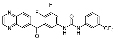
1-(3,4-difluoro-5-(quinoxaline-6-carbonyl)phenyl)-3-(3-(trifluoromethyl)phenyl)urea
