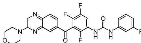
1-(3-fluorophenyl)-3-(2,4,5-trifluoro-3-(3-morpholinoquinoxaline-6-carbonyl)phenyl)urea
