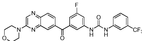
1-(3-fluoro-5-(3-morpholinoquinoxaline-6-carbonyl)phenyl)-3-(3-(trifluoromethyl)phenyl)urea
