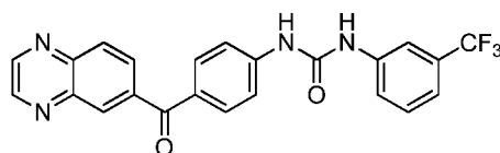
1-(4-(quinoxaline-6-carbonyl)phenyl)-3-(3-(trifluoromethyl)phenyl)urea
