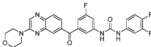
1-(3,4-difluorophenyl)-3-(3-fluoro-5-(3-morpholinoquinoxaline-6-carbonyl)phenyl)urea
