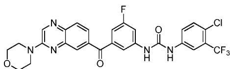
1-(4-chloro-3-(trifluoromethyl)phenyl)-3-(3-fluoro-5-(3-morpholinoquinoxaline-6-carbonyl)phenyl)urea
