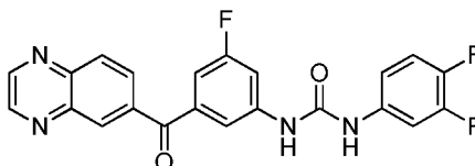
1-(3,4-difluorophenyl)-3-(3-fluoro-5-(quinoxaline-6-carbonyl)phenyl)urea
