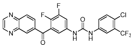
1-(4-chloro-3-(trifluoromethyl)phenyl)-3-(3,4-difluoro-5-(quinoxaline-6-carbonyl)phenyl)urea
