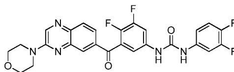
1-(3,4-difluoro-5-(3-morpholinoquinoxaline-6-carbonyl)phenyl)-3-(3,4-difluorophenyl)urea
