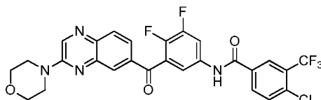
4-chloro-N-(3,4-difluoro-5-(3-morpholinoquinoxaline-6-carbonyl)phenyl)-3-(trifluoromethyl)benzamide
