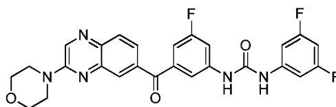
1-(3,5-difluorophenyl)-3-(3-fluoro-5-(3-morpholinoquinoxaline-6-carbonyl)phenyl)urea
