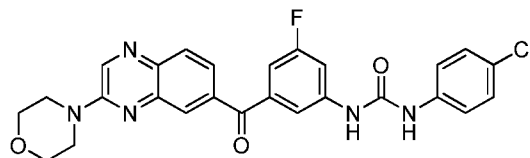
1-(4-chlorophenyl)-3-(3-fluoro-5-(3-morpholinoquinoxaline-6-carbonyl)phenyl)urea
