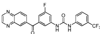
1-(3-fluoro-5-(quinoxaline-6-carbonyl)phenyl)-3-(3-(trifluoromethyl)phenyl)urea
