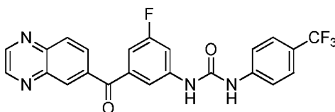
1-(3-fluoro-5-(quinoxaline-6-carbonyl)phenyl)-3-(4-(trifluoromethyl)phenyl)urea
