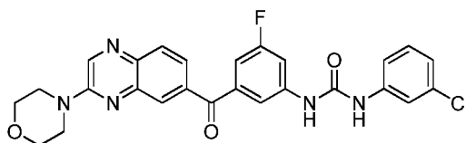
1-(3-chlorophenyl)-3-(3-fluoro-5-(3-morpholinoquinoxaline-6-carbonyl)phenyl)urea
