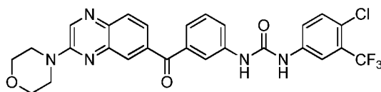
1-(4-chloro-3-(trifluoromethyl)phenyl)-3-(3-(3-morpholinoquinoxaline-6-carbonyl)phenyl)urea
