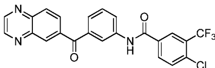
4-chloro- N -(3-(quinoxaline-6-carbonyl)phenyl)-3-(trifluoromethyl)benzamide
