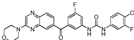
1-(4-chloro-3-fluorophenyl)-3-(3-fluoro-5-(3-morpholinoquinoxaline-6-carbonyl)phenyl)urea
