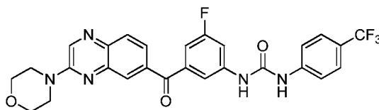
1-(3-fluoro-5-(3-morpholinoquinoxaline-6-carbonyl)phenyl)-3-(4-(trifluoromethyl)phenyl)urea
