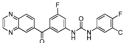
1-(3-chloro-4-fluorophenyl)-3-(3-fluoro-5-(quinoxaline-6-carbonyl)phenyl)urea
