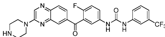
1-(4-fluoro-3-(3-(piperazin-1-yl)quinoxaline-6-carbonyl)phenyl)-3-(3-(trifluoromethyl)phenyl)urea
