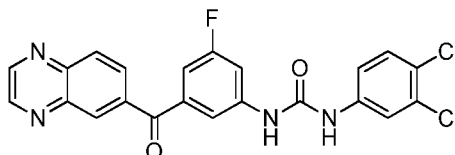
1-(3,4-dichlorophenyl)-3-(3-fluoro-5-(quinoxaline-6-carbonyl)phenyl)urea
