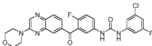
1-(3-chloro-5-fluorophenyl)-3-(4-fluoro-3-(3-morpholinoquinoxaline-6-carbonyl)phenyl)urea
