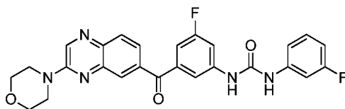
1-(3-fluoro-5-(3-morpholinoquinoxaline-6-carbonyl)phenyl)-3-(3-fluorophenyl)urea
