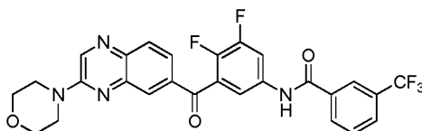
N-(3,4-difluoro-5-(3-morpholinoquinoxaline-6-carbonyl)phenyl)-3-(trifluoromethyl)benzamide
