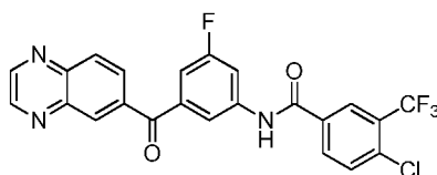
4-chloro-N-(3-fluoro-5-(quinoxaline-6-carbonyl)phenyl)-3-(trifluoromethyl)benzamide
