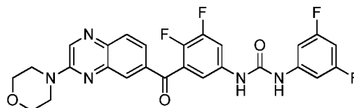
1-(3,4-difluoro-5-(3-morpholinoquinoxaline-6-carbonyl)phenyl)-3-(3,5-difluorophenyl)urea
