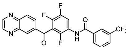
N -(2,4,5-trifluoro-3-(quinoxaline-6-carbonyl)phenyl)-3-(trifluoromethyl)benzamide
