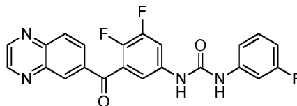
1-(3,4-difluoro-5-(quinoxaline-6-carbonyl)phenyl)-3-(3-fluorophenyl)urea
