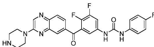
1-(3,4-difluoro-5-(3-(piperazin-1-yl)quinoxaline-6-carbonyl)phenyl)-3-(4-fluorophenyl)urea
