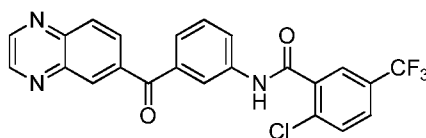
2-chloro-N-(3-(quinoxaline-6-carbonyl)phenyl)-5-(trifluoromethyl)benzamide
