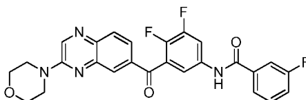
N-(3,4-difluoro-5-(3-morpholinoquinoxaline-6-carbonyl)phenyl)-3-fluorobenzamide
