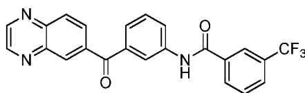
N -(3-(quinoxaline-6-carbonyl)phenyl)-3-(trifluoromethyl)benzamide
