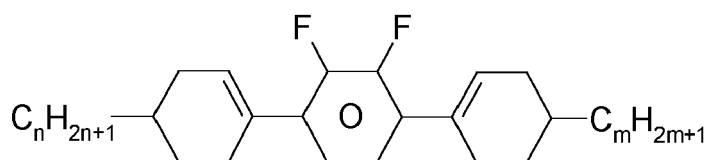
LYLI-n-m
