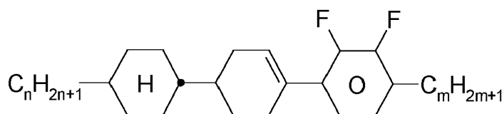
CLY-n-m
