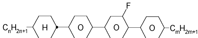
CPGP-n-m
