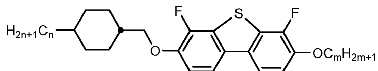
COB(S)-n-Om
