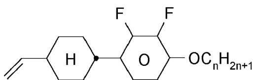
CY-V-On
