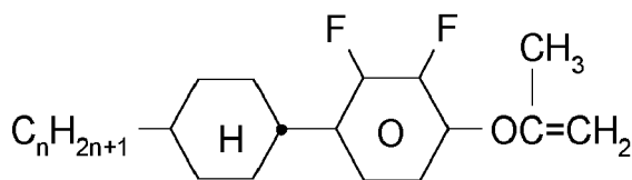
CY-n-OC(CH 3 )=CH 2
