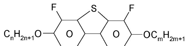
B(S)-nO-Om
