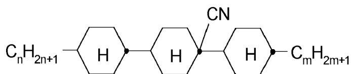
BCN-nm
