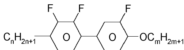
YG-n-Om
