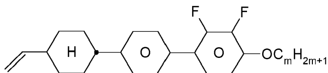
CPY-V-Om
