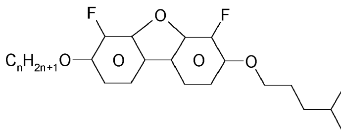
B-nO-O5i
