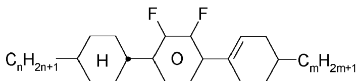
CYLI-n-m
