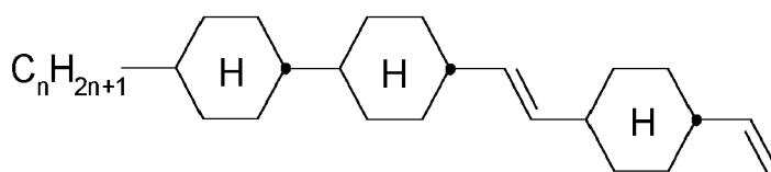
CCVC-n-V
