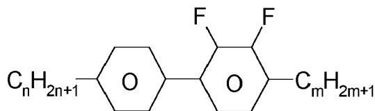
PY-n-m
