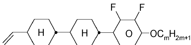
CCY-V-Om
