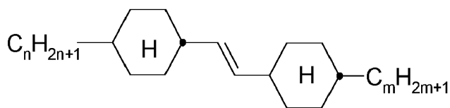
CVC-n-m
