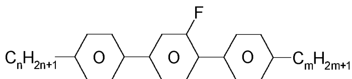
PGP-n-m
