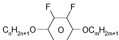
Y-nO-Om
