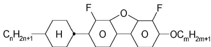
CB-n-Om
