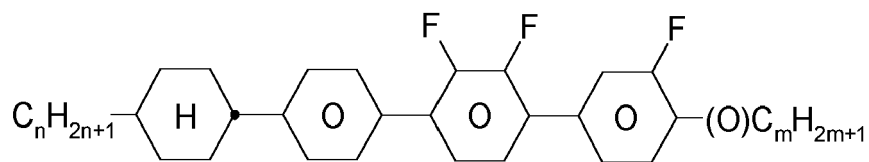
CPYG-n-(O)m
