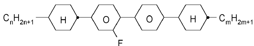
CBC-nmF
