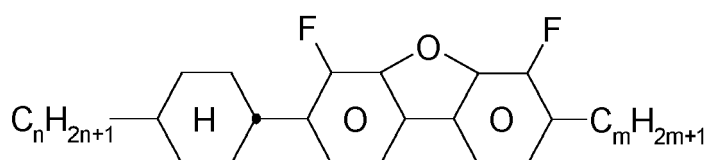
CB-n-m
