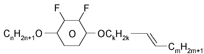
Y-nO-OkVm
