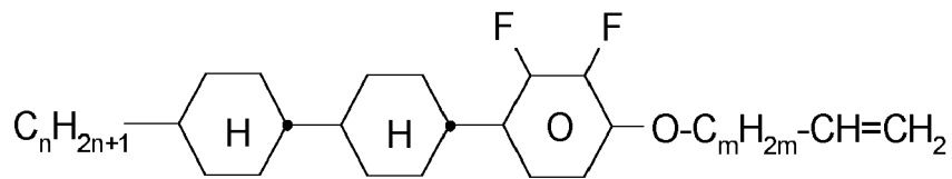
CCY-n-OmV
