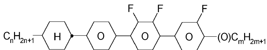
CPYG-n-(O)m
