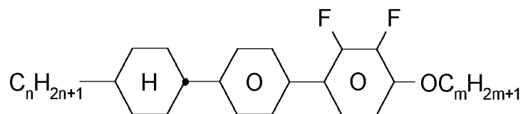
CPY-n-Om
