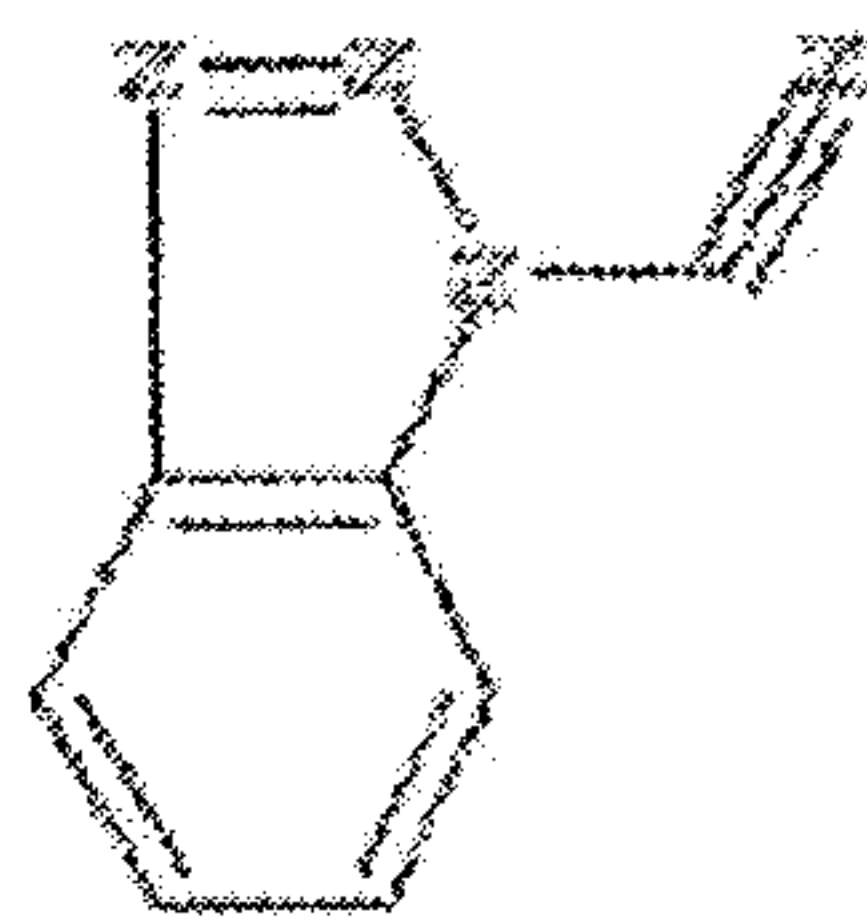
1-cyanobenzotriazole (1-CBT)
