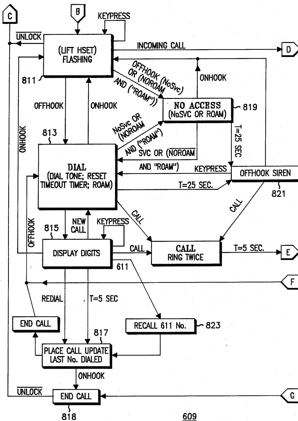
FIG. 8B
