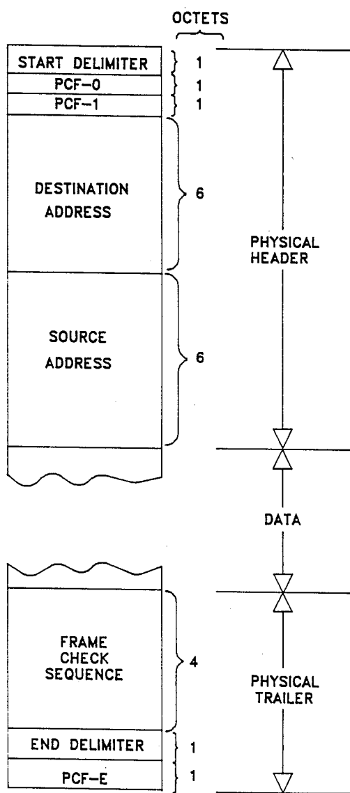
FIG. 3 FRAME FORMAT
