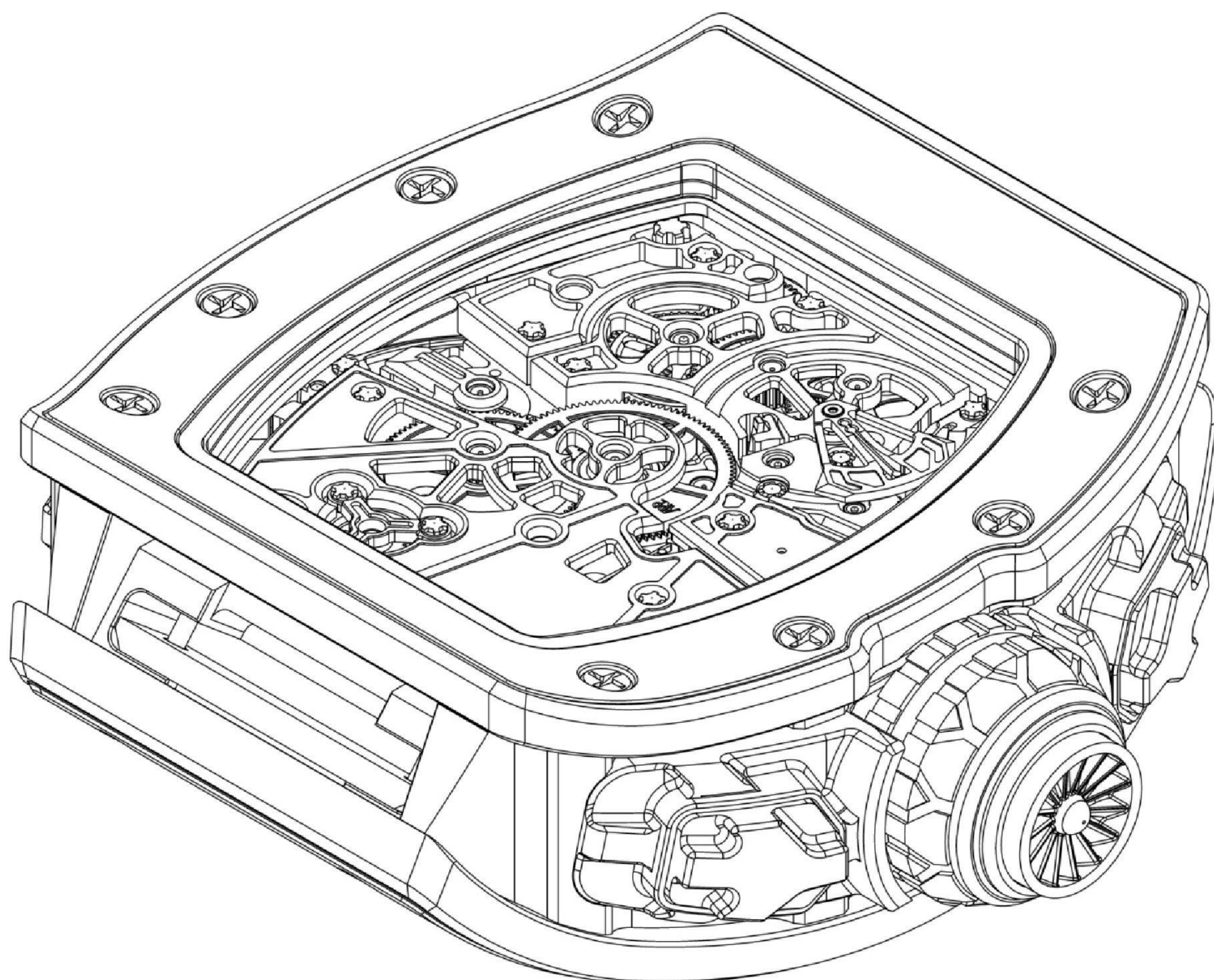
【立體圖4】
