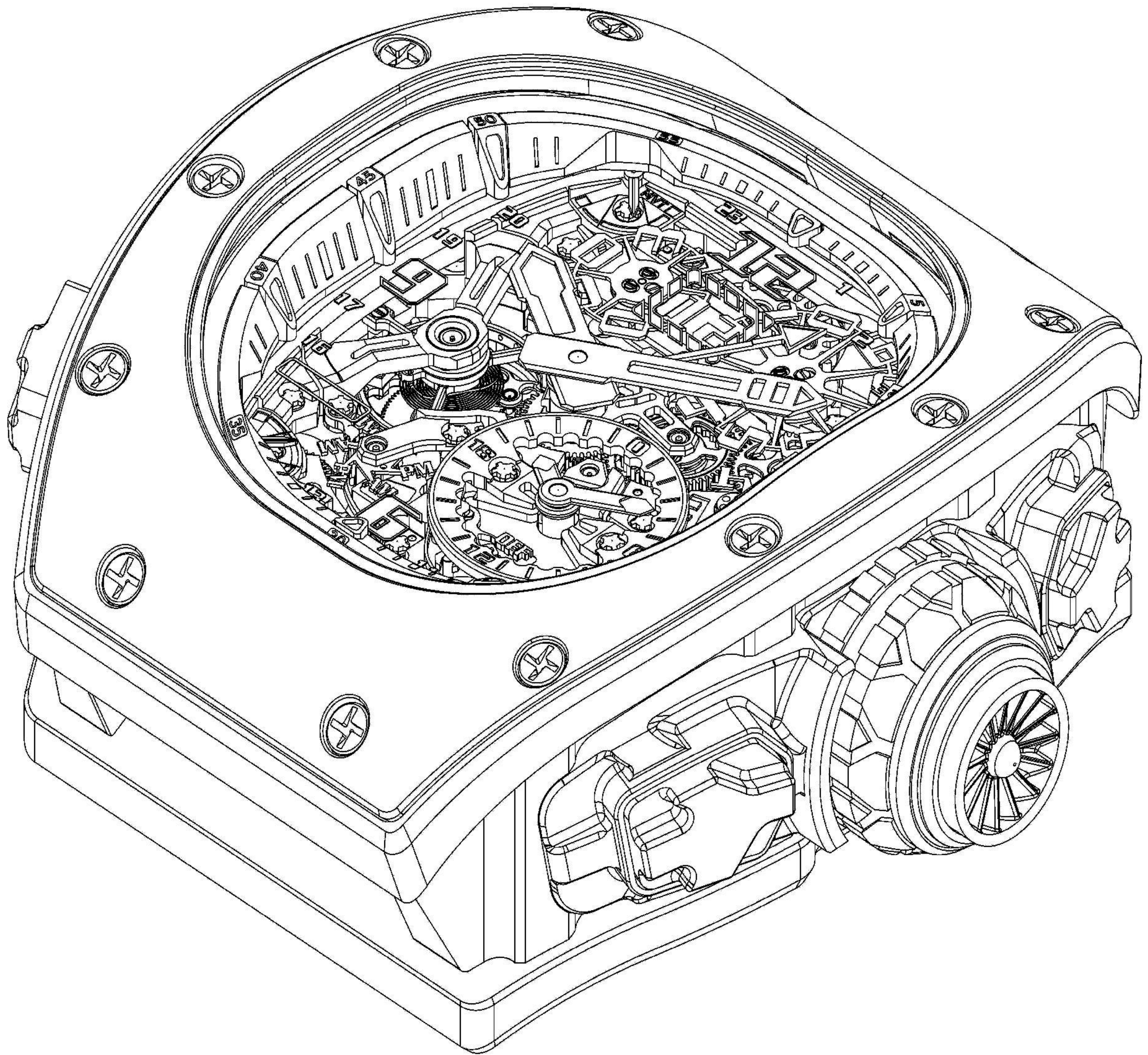
【立體圖1】
